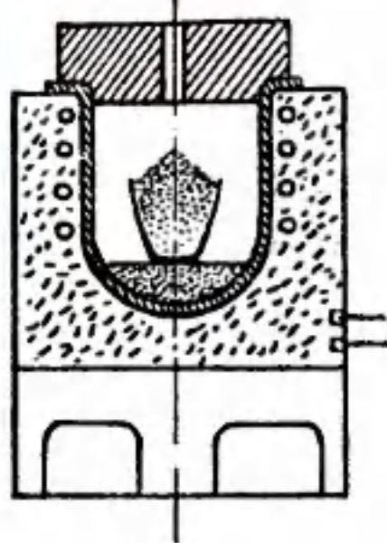
Поперечный разрез лабораторной тигельной печи.
